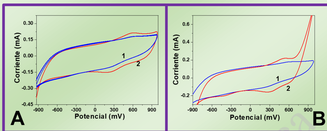
Figura 1: Voltamperogramas cíclicos para (A) SPE- desnudo y (B) SPE- ionóforo, en (1) \text{H}_2\text{SO}_4 pH: 1,0 y (2) \text{Cr(VI)} 0,2 mM en \text{H}_2\text{SO}_4 pH: 1,0. Los barridos se realizaron desde 1000 mV hasta -1000 mV para volver finalmente al potencial inicial. Velocidad de barrido: 50 \text{ mVs}^{-1} . Electrodo de referencia: \text{Ag/AgCl} . Contraelectrodo: Platino.
