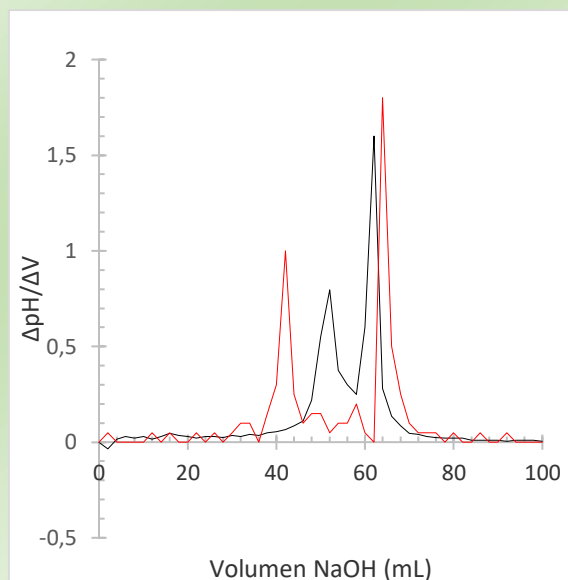
Figura 6. Determinación de grupos \text{NH}_2 del \text{Qhl}_{11} y \text{Qhc} .
