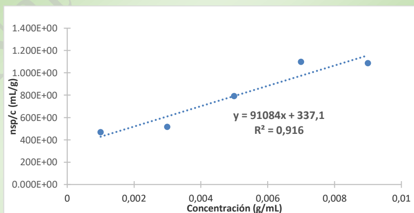
Figura 4. Gráfica de viscosidad reducida en función de la concentración en masa de las soluciones de quitosán para determinar el Mv de Qhl 11 por viscosimetría.
