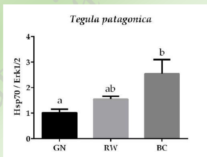
Figura 5. Niveles de expresión Hsp70 en gónada de Tegula patagonica , sobre muestras recolectadas en el IN durante las temporadas de verano e invierno en GN, RW y BC. Los graficos resumen la expresion de Hsp70 en 3-5 muestras independientes (media±DS). Letras distintas hacen referencia a diferencias significativas entre las medias de las localidades, con un p < 0,05 correspondiente a una prueba a posteriori de Tukey.
