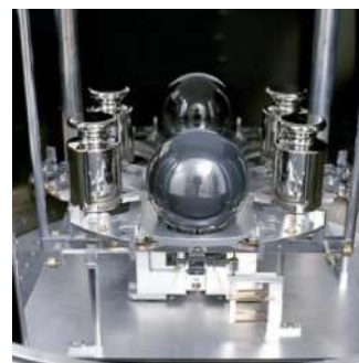
Esfera de ^{28}\text{Si} . Extraída de http://www.cem.es
