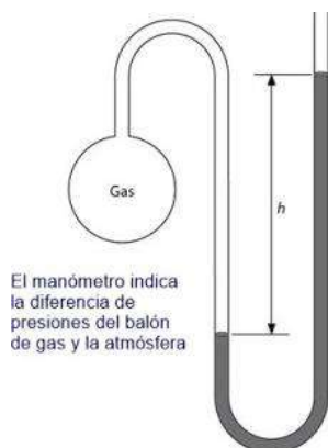
Ilustración 4. Manómetro abierto. Extraída de: http://www.instrumentosdelaboratorio.net/2014/08/manometro.html
